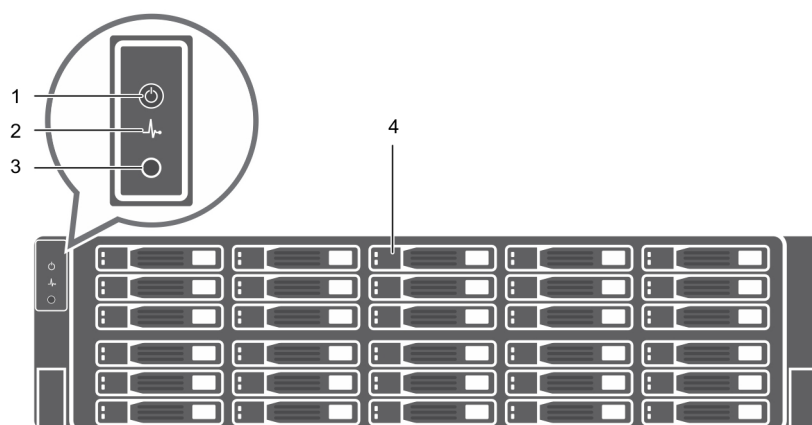
图 1: SC7020 系列存储系统前面板视图
